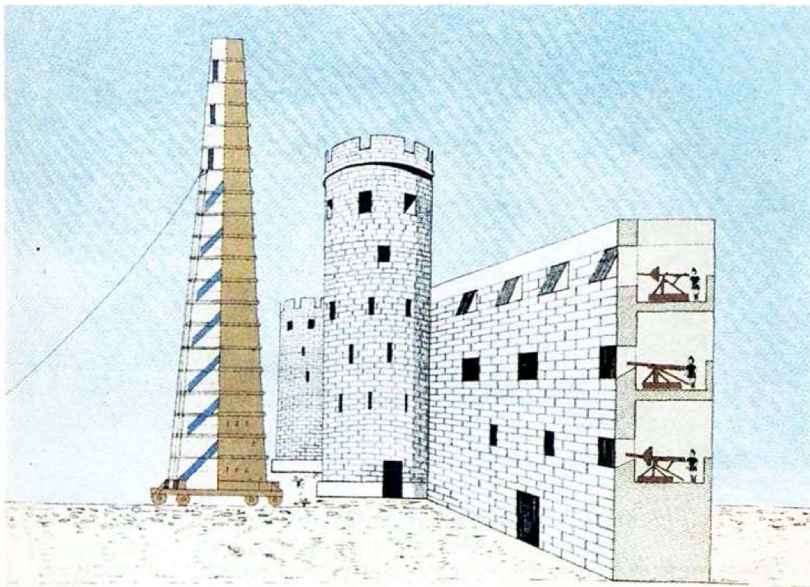
Πολιορκητικοί Πύργοι
