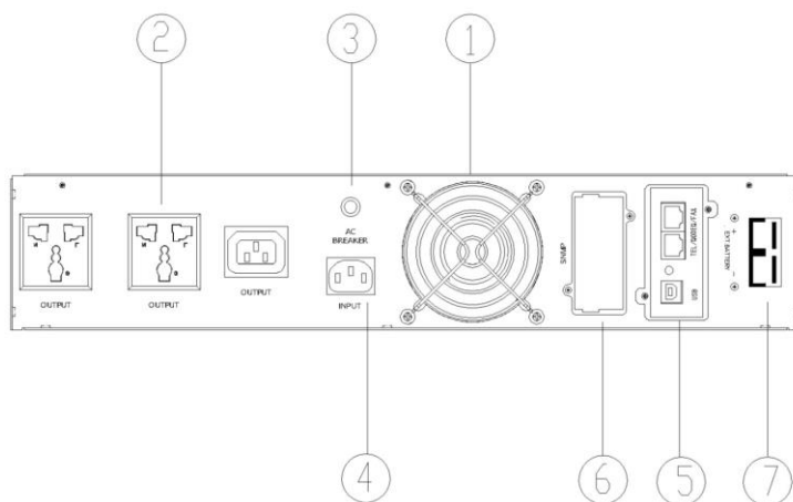
Εικόνα 2.3.2 Πίσω όψη 2U 1KVA
