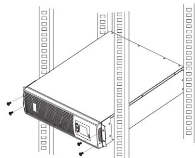
Εικόνα 2.4.3 Εγκατάσταση σε Rack
